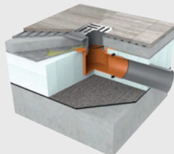
Skladba balkonu s lepenou vrstvou
