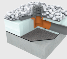
Skladba balkonu s vrstvou kačírku
