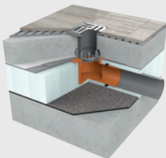
Skladba balkonu s drenážní vrstvou
