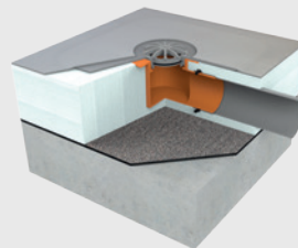
Skladba balkonu s pochozí střešní folií
